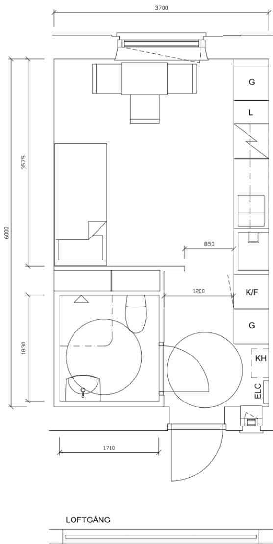
BYGGD LGH I FURIREN 20,4 KVM
