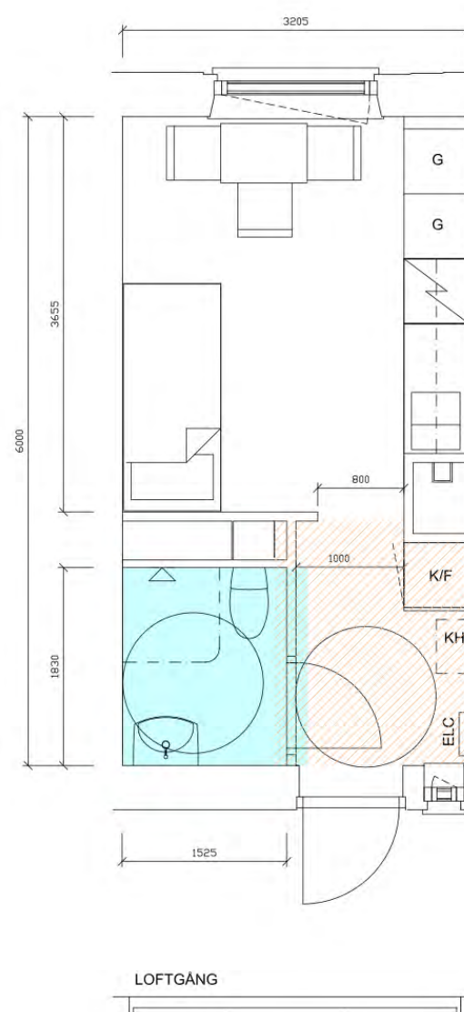
FÖRESLAGEN LGH I FURIREN 17,9 KVM ALTERNATIV B
